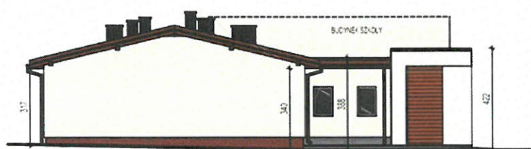
ELEWACJA ZACHODNIA
